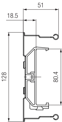
MultiLine 0831、4極
