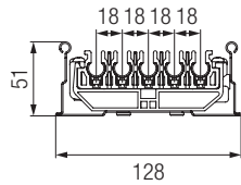
0831 4 poles
