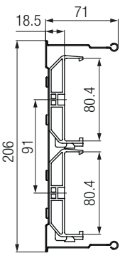
MultiLine 0831、 4+4極
