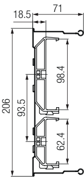
MultiLine 0831、 5+3極
