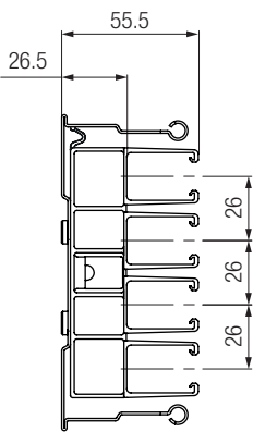
SinglePowerLine 0812、4極
