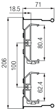
MultiLine 0831、 3+4極
