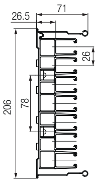
SinglePowerLine 0812、7極
