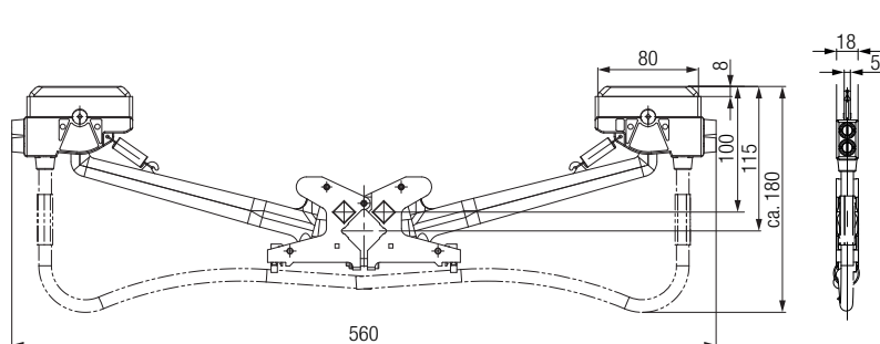
ダブルコレクタ 両方向移動用構成
