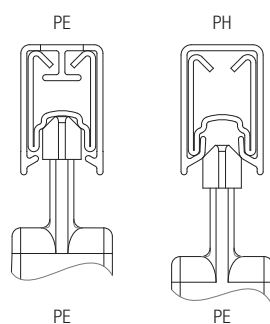
PE-PH誤接続保護
