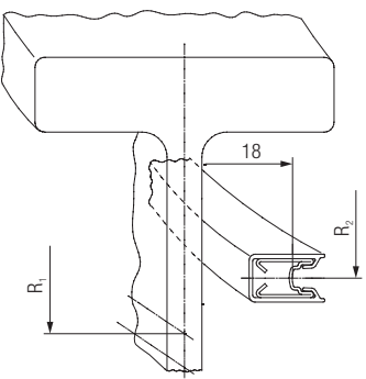
傾斜部(側方からのエントリー)
