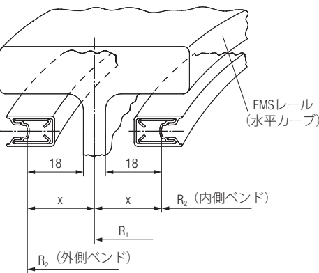
コンダクターレールカーブ(側方からのエントリー)
