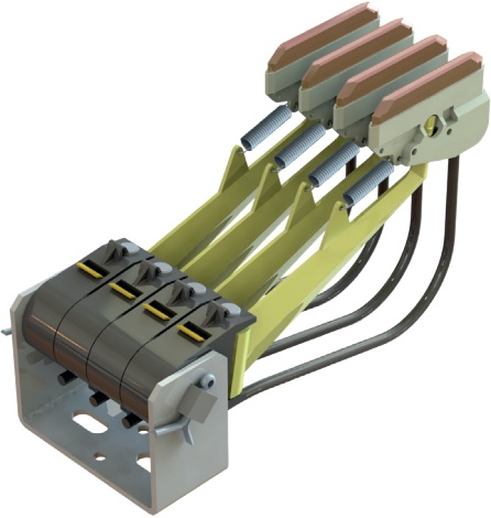
コンダクターレールの極番号
